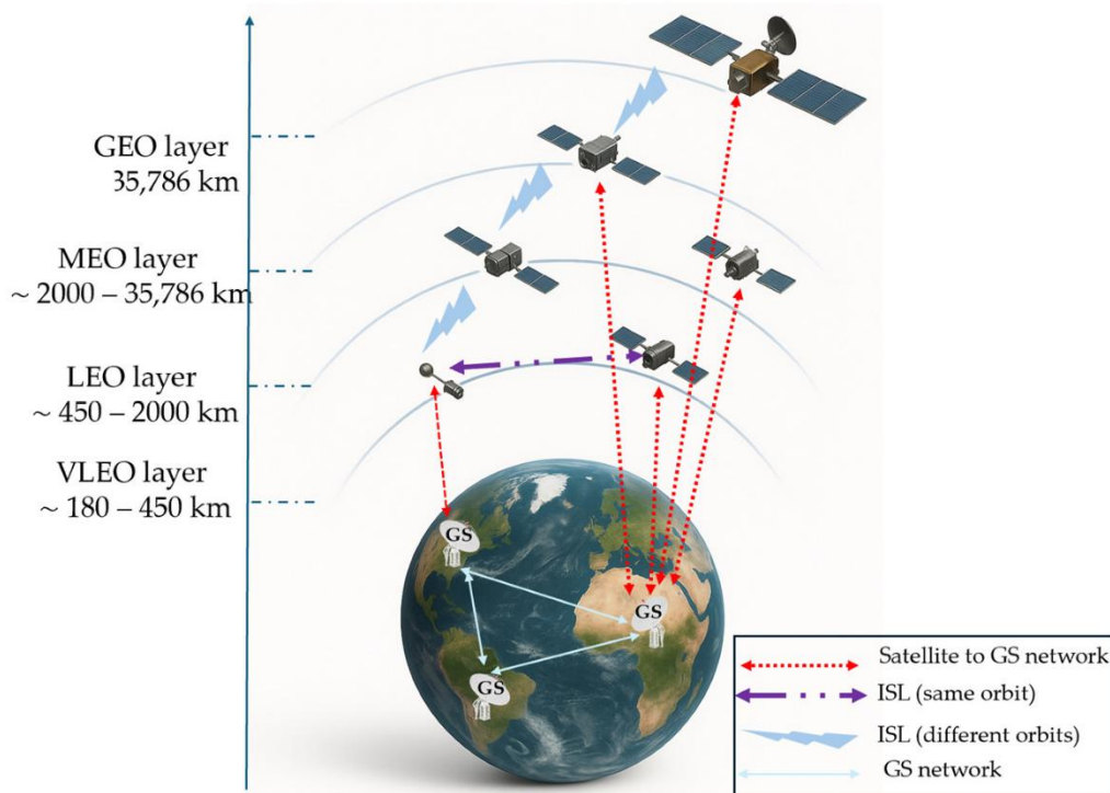
圖一：各軌道衛星高度示意圖
